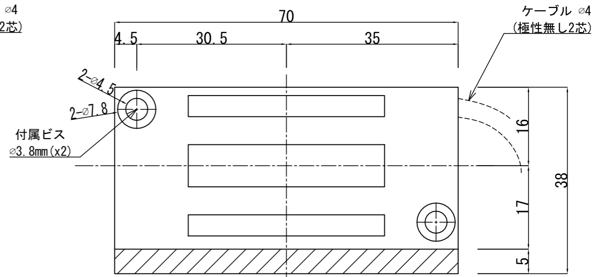
本体+ブラケット 正面図
