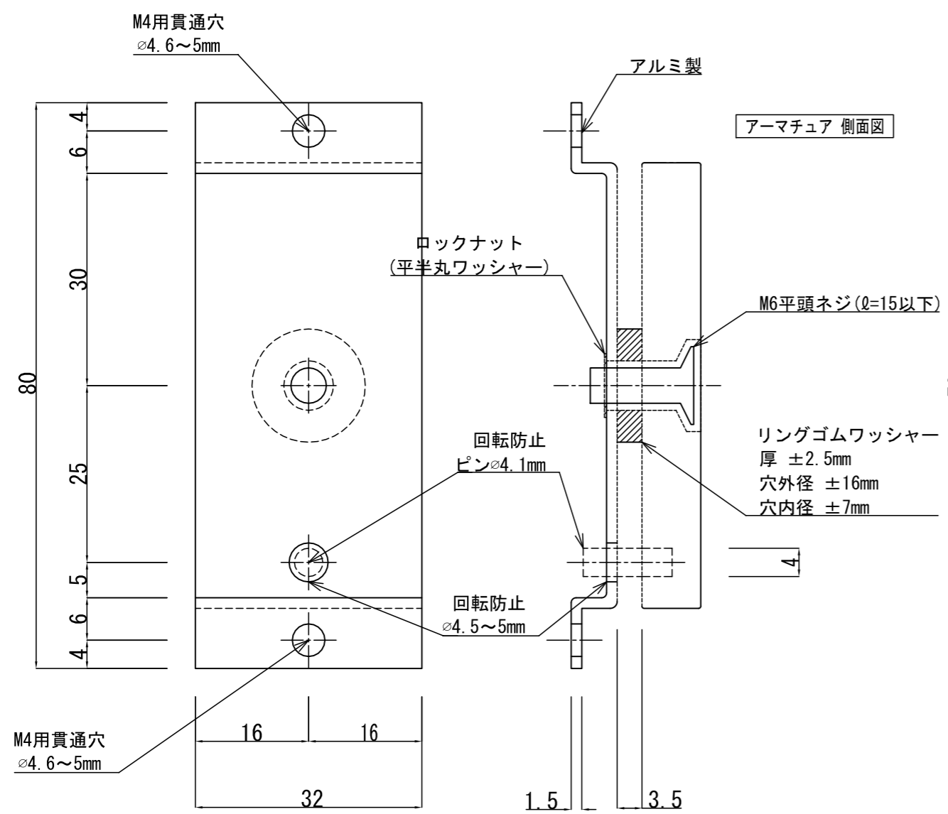
アーマチュア 裏面図
