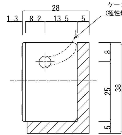
本体+ブラケット 見下図
