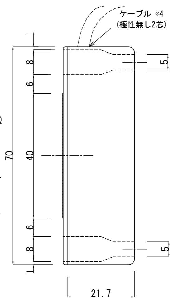
本体 側面図
