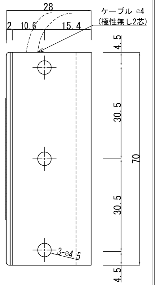
本体+ブラケット 側面図
