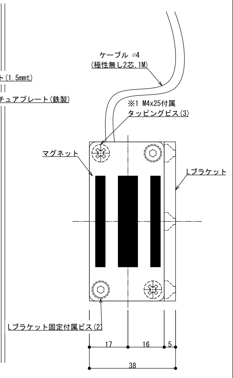
マグネット・ドアホルダー Lブラケット組品 正面図
